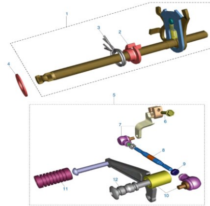
Figura N° 9: Mecanismo de cambios
