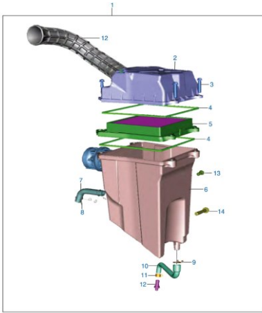
Figura N° 19: Filtro de aire
