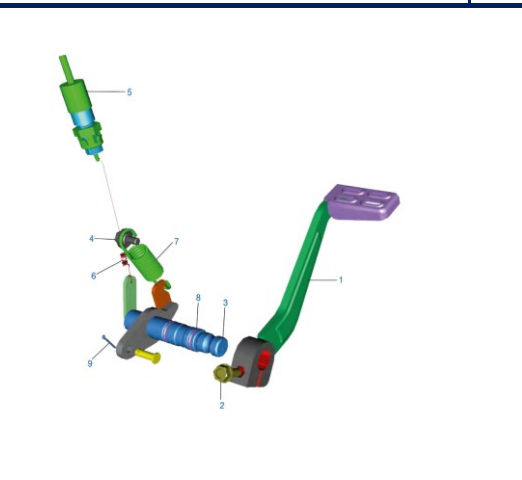
Figura N° 36: Pedal de freno
