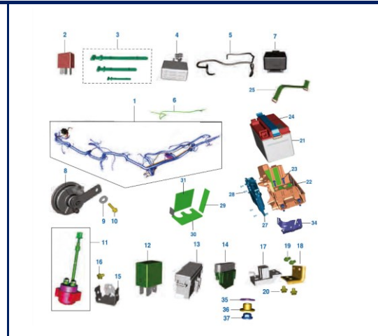
Figura N° 51: Sistema Electrico
