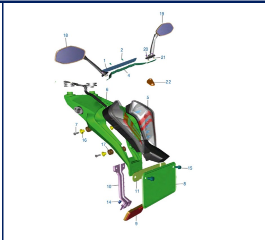
Figura N° 50: Stop Completo
