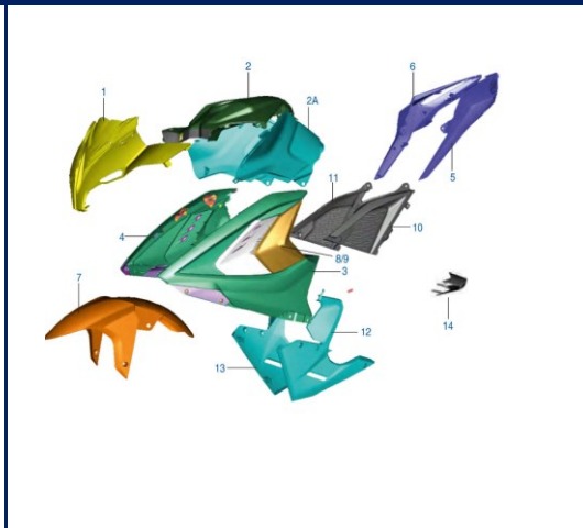
Figura N° 53: Cobertores
