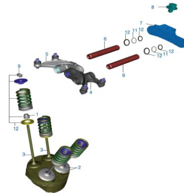
Figura N° 3: Valvulas
