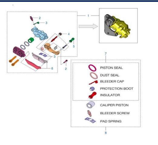
Figura N° 33: Mordaza de freno delantero
