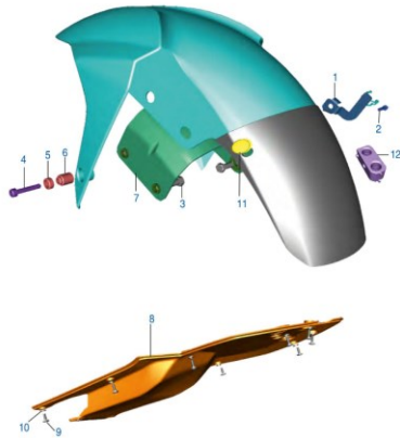
Figura N° 28: Loderas
