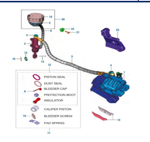
Figura N° 35: Mordaza de freno trasero
