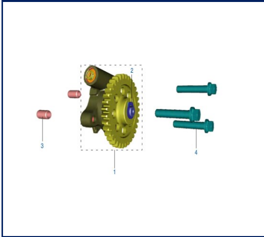
Figura N° 13: Bomba de aceite
