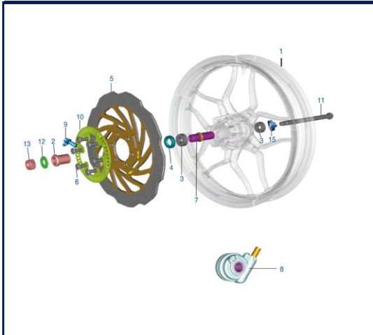
Figura N° 31: Freno delantero
