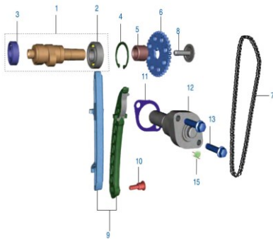
Figura N° 4: Eje de levas y tensor de cadena
