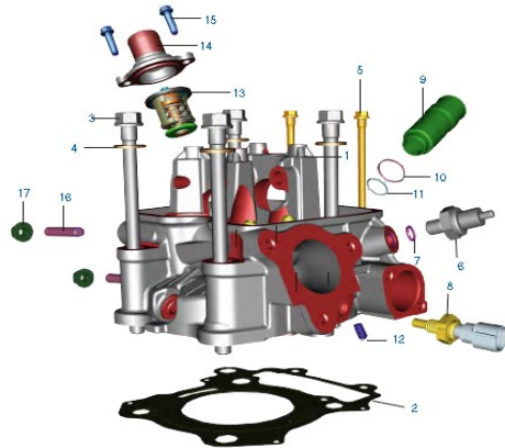
Figura N° 2: Culata
