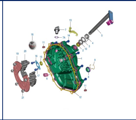
Figura N° 15: Tapadera de clutch
