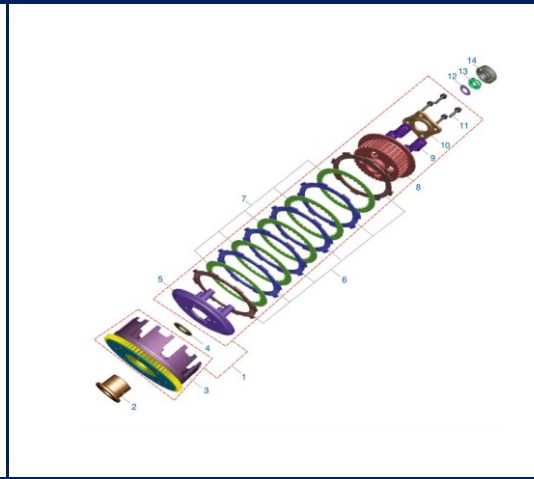
Figura N° 17: Clutch
