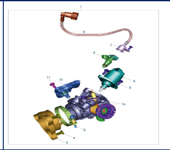
Figura N° 18: Inyector
