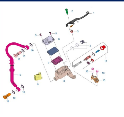
Figura N° 32: Bomba de freno
