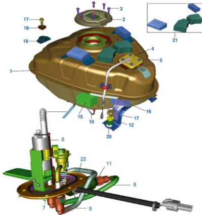
Figura N° 40: Tanque de combustible
