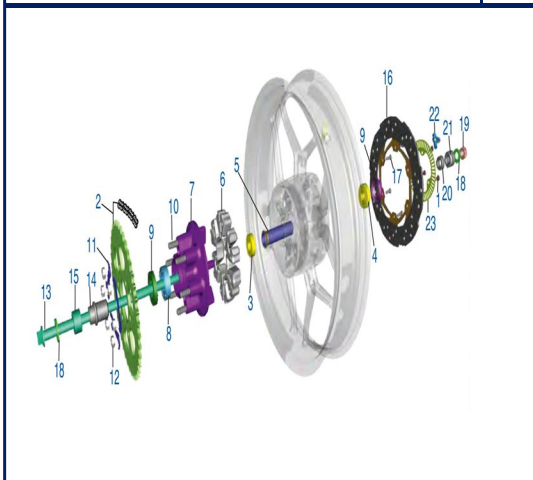
Figura N° 34: Masa trasera
