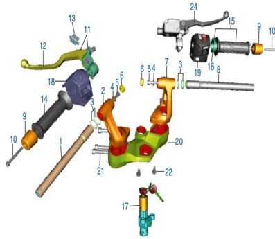
Figura N° 38: Controles
