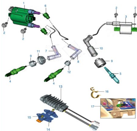
Figura N° 22: Bobina HT
