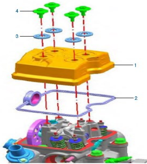
Figura N° 1: Tapadera de culata
