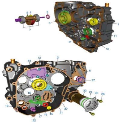
Figura N° 10: Carter RH
