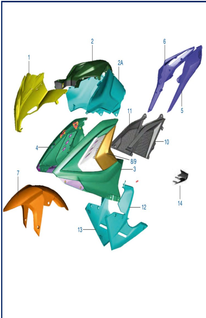
FIGURA N°53: COBERTORES
