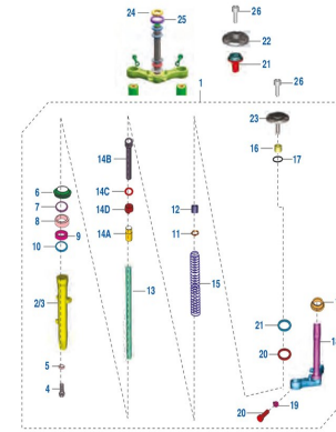
Figura N° 39: Tren Delantero
