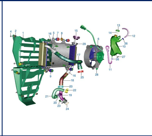
Figura N° 14: Radiador
