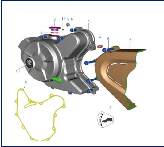
Figura N° 16: Cobertor de magneto
