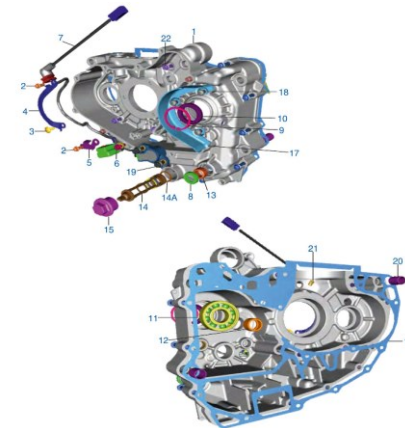
Figura N° 11: Tapadera de carter LH
