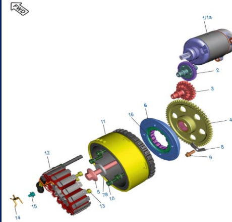
Figura N° 21: Estarter
